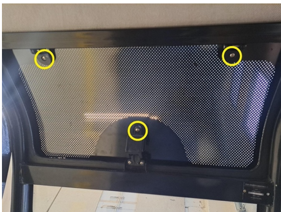
Irrota kattoluukun kiinnitysruuvit. (ristipäämeisseli ph2).
